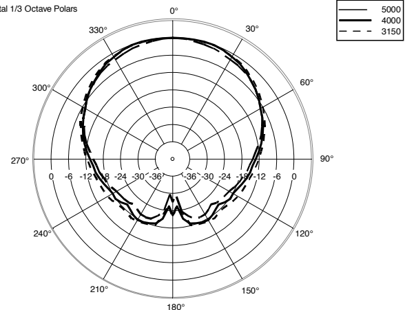
Horizontal 1/3 Octave Polars
