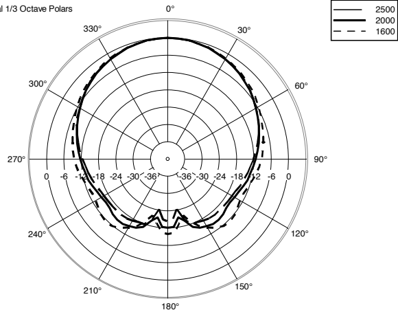
Horizontal 1/3 Octave Polars
